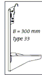
type 33, 300 mm a : 199 mm b : 78 mm c : 25 mm
