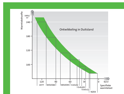
Afb. A.2 Warmtebehoefte in een ruimte – specifiek warmtelastdiagram voor schattingsdoeleinden
