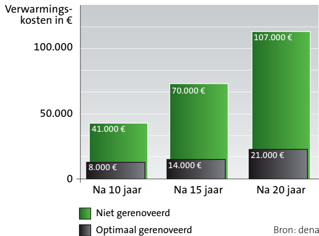
Afb. 2.1 Geschatte verwarmingskosten voor een eengezinswoning: met en zonder isolatie
