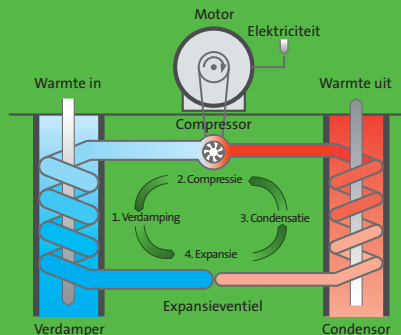
Afb. 3.1 Diagram van een warmtepomp
