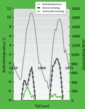
Externe warmtewinsten 17-18 maart - weergegevens
