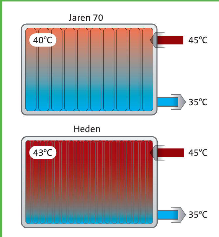
Afb. 1.3 Innovatie in paneelradiatoren
