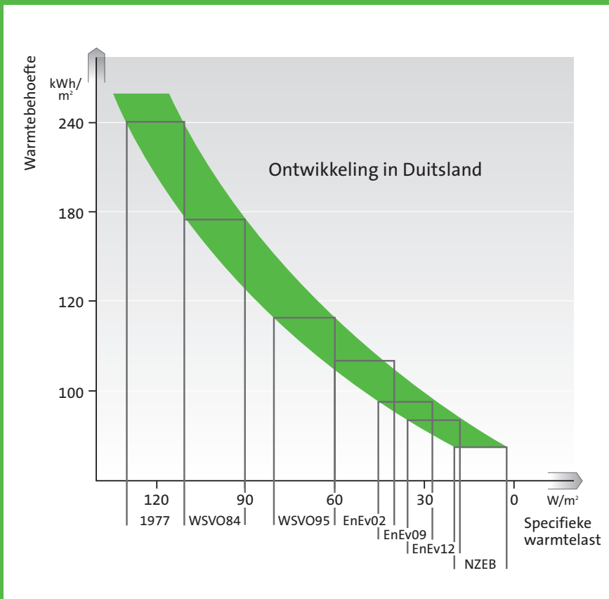
Afb. 3.9 Ruimteverwarming s-behoeft -specifieke warmtelast- diagram voor schattings- doeleinden
