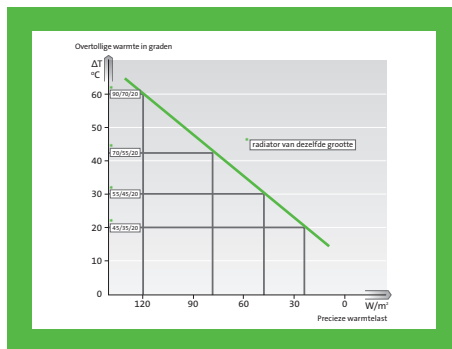
Afb. A.1 Radiatorkwerktemperaturen zijn omlaag gegaan in samenhang met de gedaalde warmtelast van gebouwen
