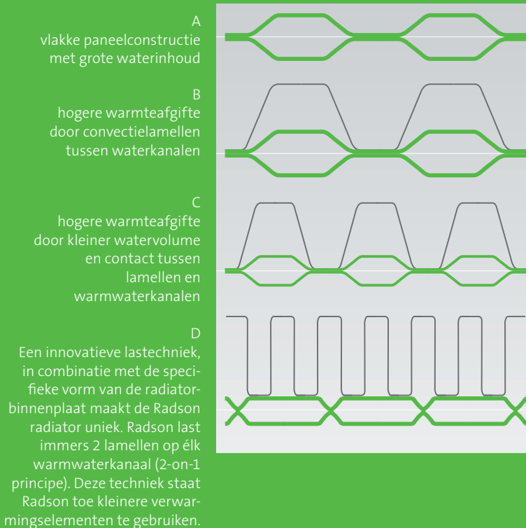
Afb. 1.2 Innovatie in paneelradiatoren
