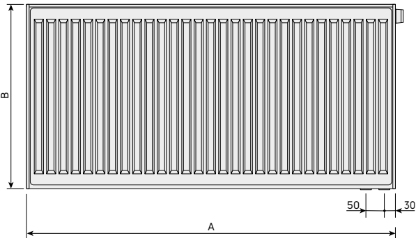
Vue avant
