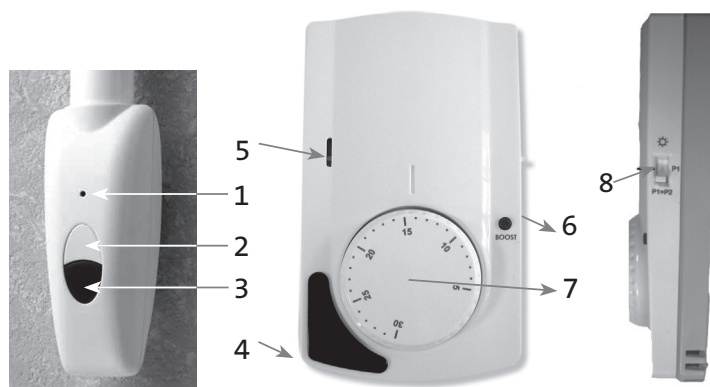
Infrarot-Empfänger Analoger Infrarot-Raumthermostat
